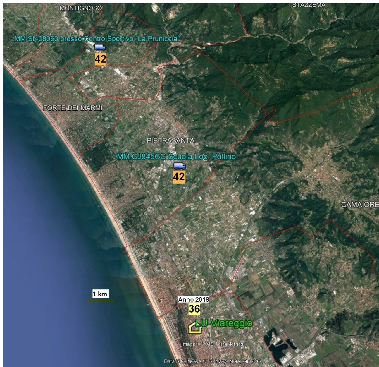
Figura 5.2.3.b – Mappa con i valori relativi al 90,4°percentile, espressi in \mu\text{g}/\text{m}^3 , nei vari siti di misura. Per LU-Viareggio è stato considerato l'indicatore 90,4° percentile su tutti i dati di PM10 riferiti al 2018.
