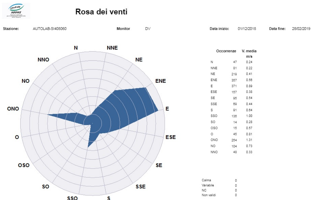
Grafico A.1.3 Rosa dei venti, Strettoia - "La Pruniccia" - inverno 2018/2019
