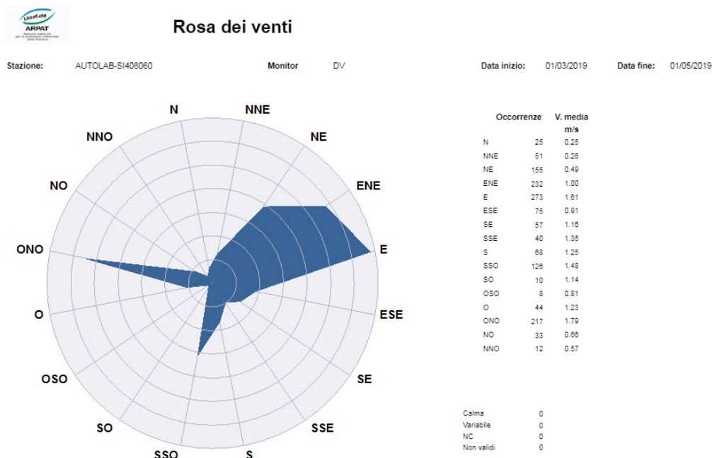
Grafico A.1.4 Rosa dei venti, Strettoia - "La Pruniccia" - primavera 2019
