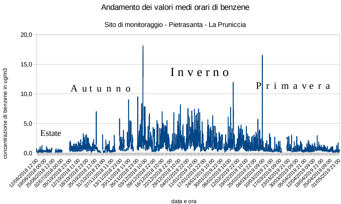
Grafico 5.2.6.1 – andamento dei valori medi orari di benzene misurato alla Pruniccia nelle varie stagioni
