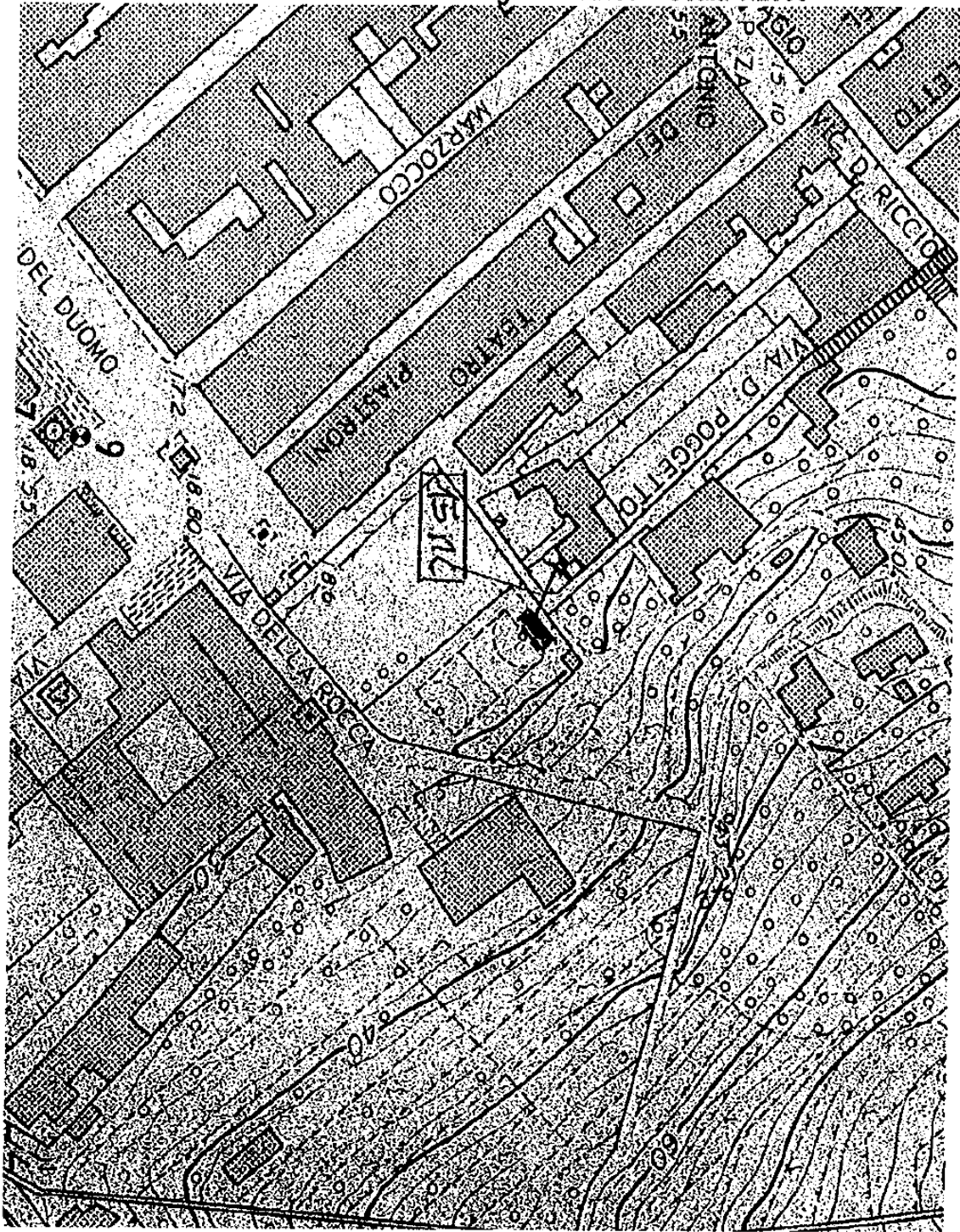
Planimetria estratto aerofotogrammetrico – Scala 1:2000
